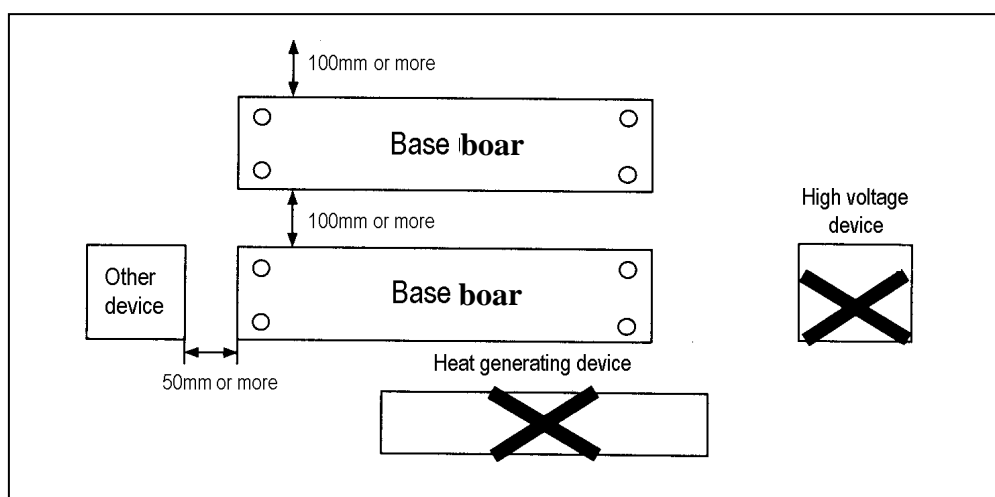
[Fig. 10.1] PLC
